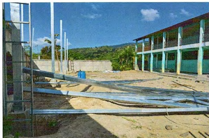
Foto 3: Durante a mejoramiento de las bases de concreto y vigas de metal
